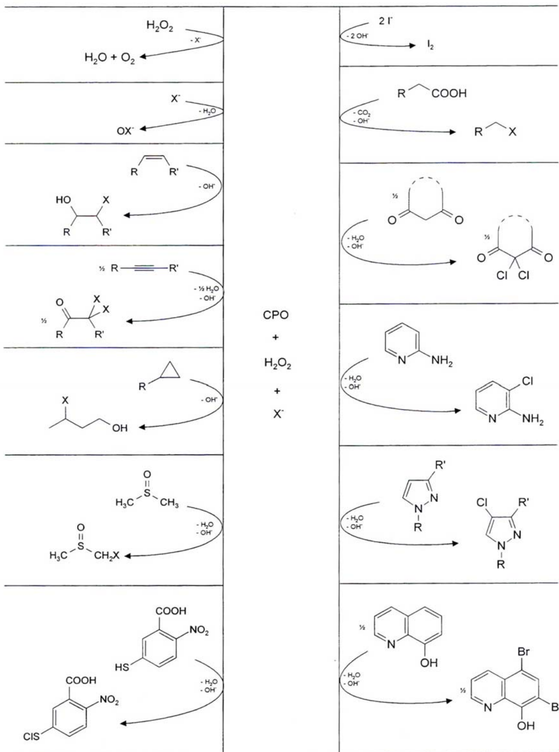
Abb. 2: Schemata der Chloroperoxidase-katalysierten Reaktionen unter Anwesenheit von Halogenidionen
